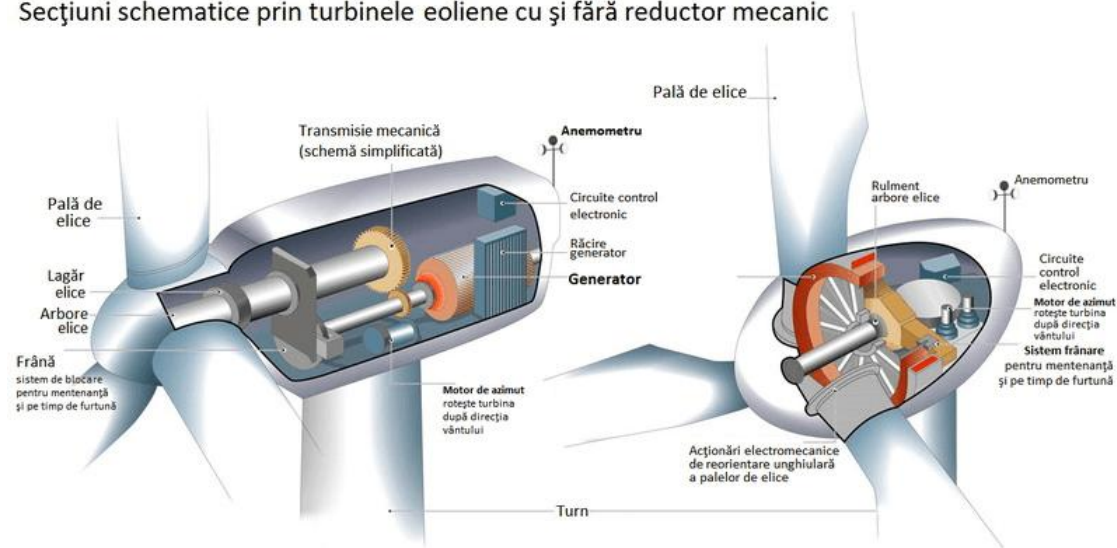
Secțiuni schematice prin turbinele eoliene cu și fără reductor mecanic
